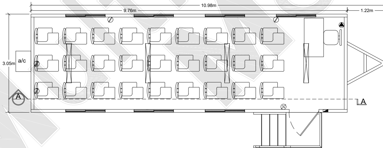
MM1036 AULA 18 A 33 PERSONAS Esc. 1:70
