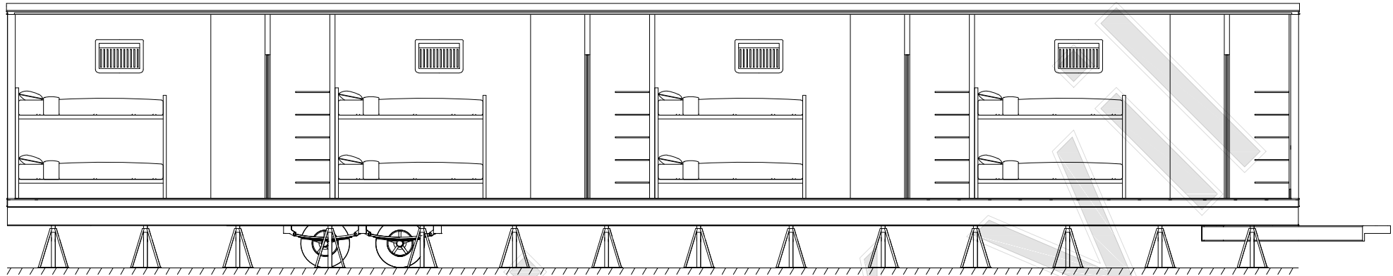
SECCIÓN A-A Esc.1:70
