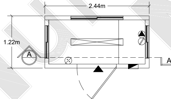
MM48 Esc.1:50
