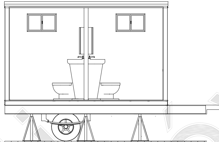
SECCIÓN A-A Esc. 1:50
