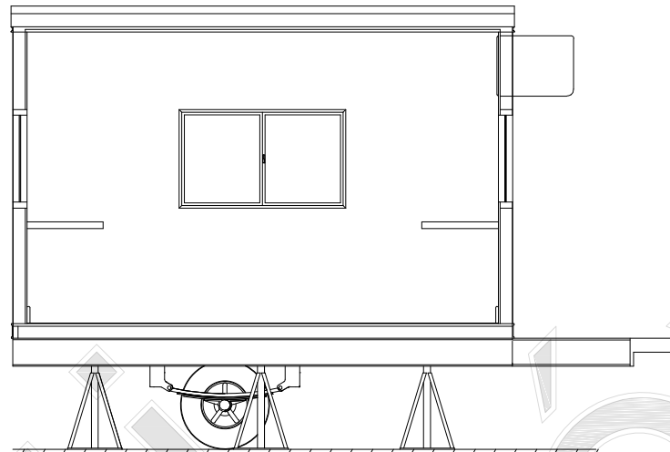
SECCIÓN A-A Esc. 1:50
