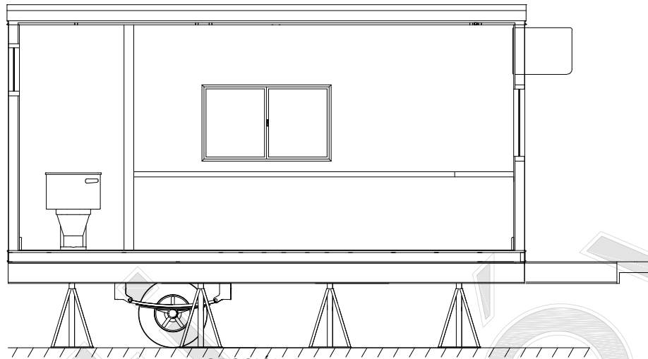
SECCIÓN A-A Esc.1:50
