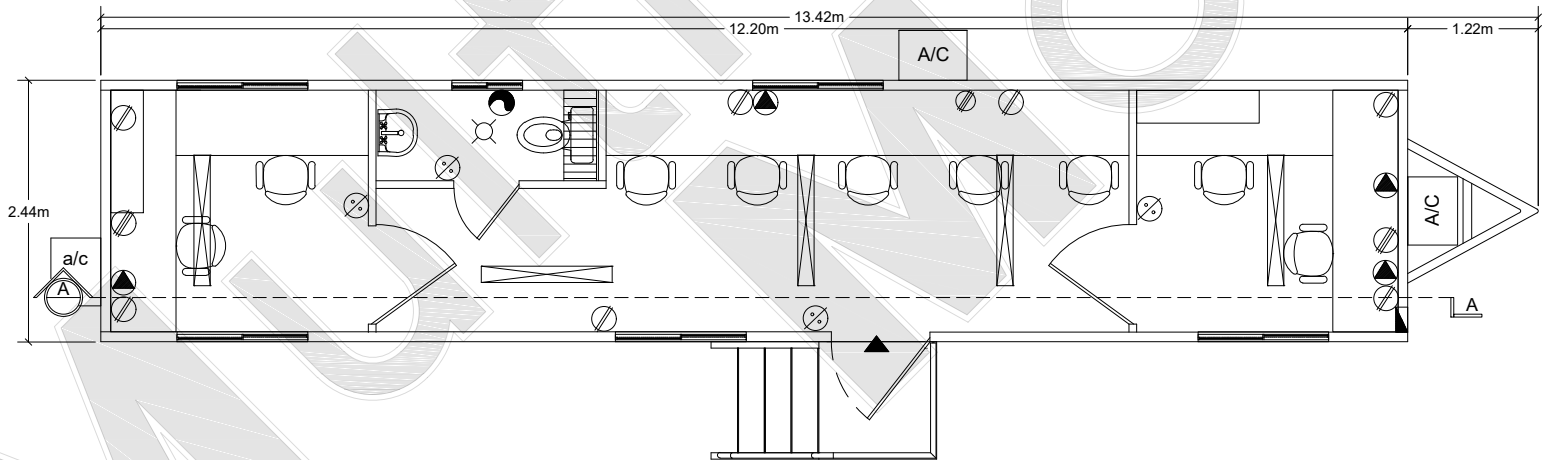
MMB844 7 A 9 PERSONAS Esc. 1:70
